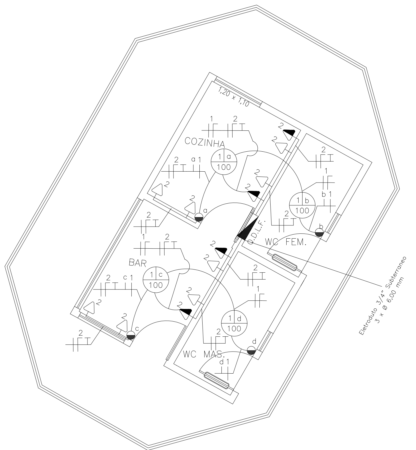
Planta Eléctrica Escala 1:50
